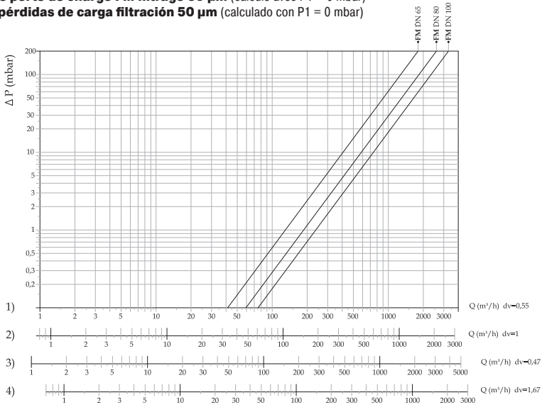
Diagramma perdite di carico FM filtraggio 50 µm (calcolato con P1 = 0 mbar) FM pressure drop diagram filtering 50 µm (calculated with P1 = 0 mbar) Diagramme de perte de charge FM filtrage 50 µm (calculé avec P1 = 0 mbar) Diagrama de pérdidas de carga filtración 50 µm (calculado con P1 = 0 mbar)
