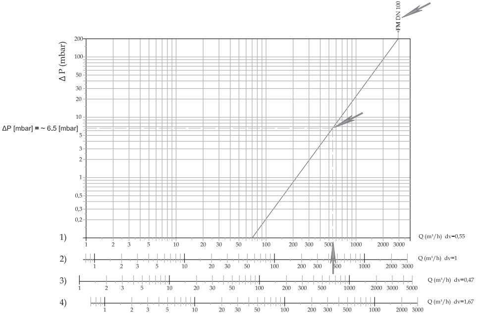
Diagramma perdite di carico FM filtraggio 50 µm (calcolato con P1 = 0 mbar) FM pressure drop diagram filtering 50 µm (calculated with P1 = 0 mbar) Diagramme de perte de charge FM filtrage 50 µm (calculé avec P1 = 0 mbar) Diagrama de pérdidas de carga filtración 50 µm (calculado con P1 = 0 mbar)
